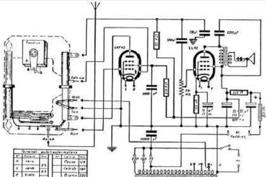
Schema elettrico *GNOMO* RICEV. R 2
