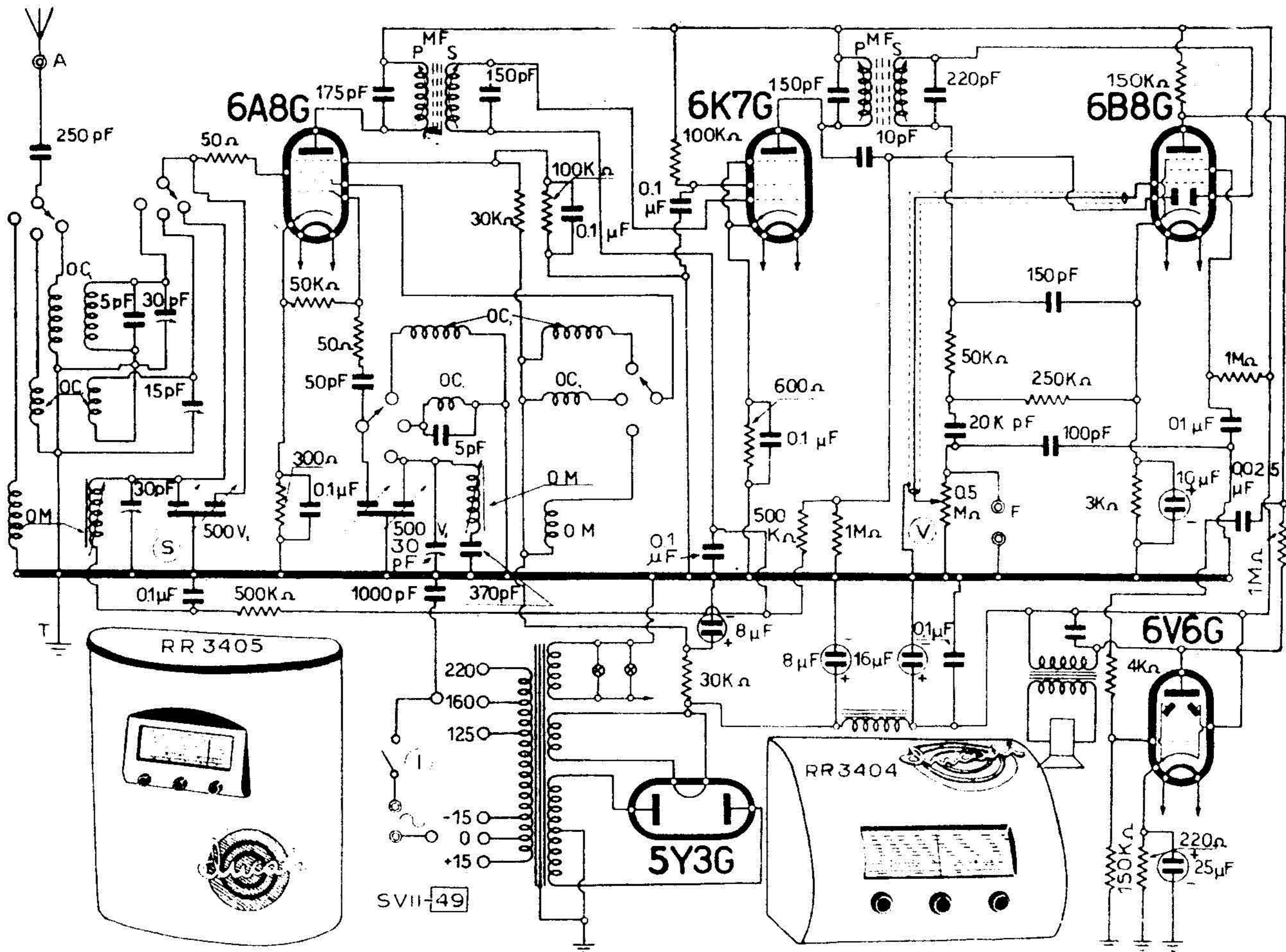
DUCATI - MODD. « RR 3404 » « RR 3405 FONO »
