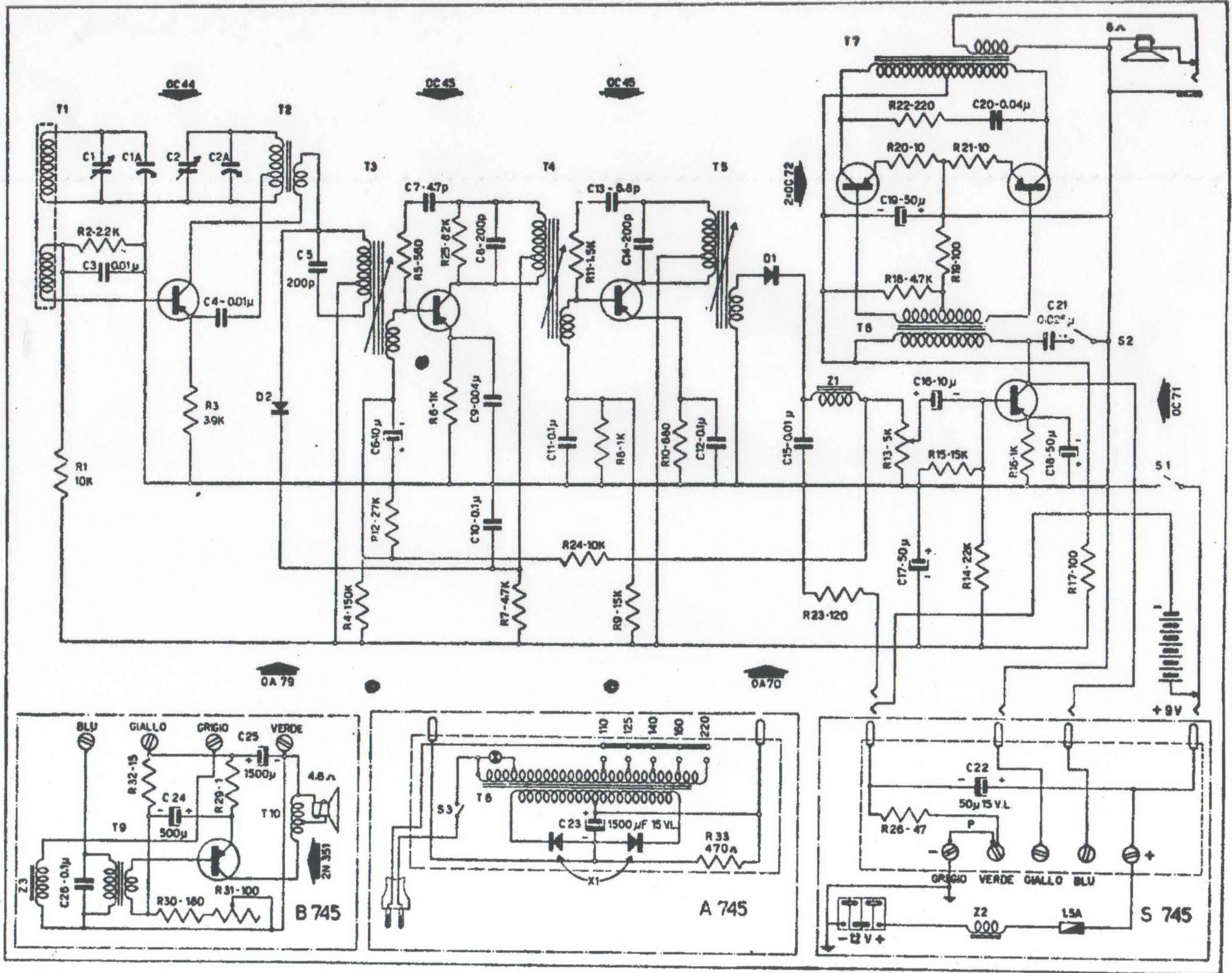
SCHEMA ELETTRICO 745. 1-5513
