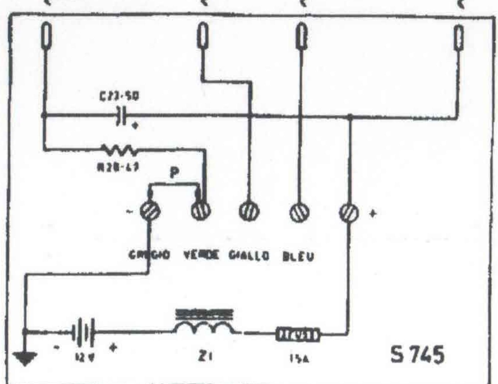
Schema elettrico del radioricevitore VOXSON mod. 752 Zephir 30
