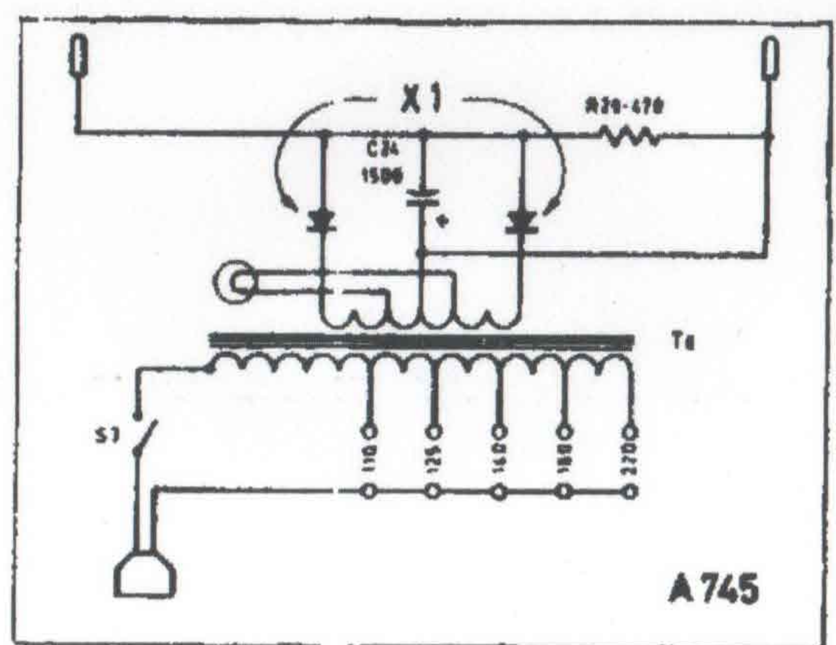
Schema elettrico del radioricevitore VOXSON mod. 752 Zephir 30
